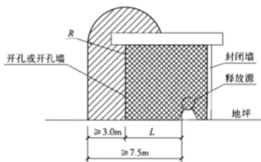
图 C.0.13 CNG 压缩机、阀门、法兰或类似附件的房间爆炸危险区域划分
