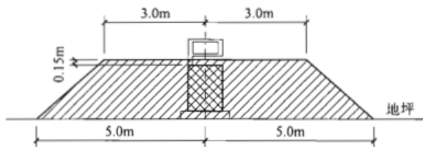
图 C.0.7 LPG 加气机的爆炸危险区域划分
