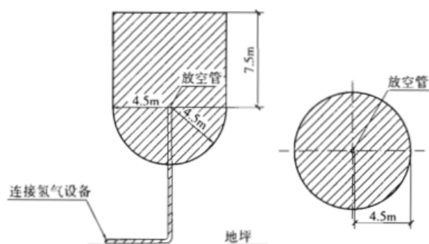
图 C.0.23 氢气设备放空管的爆炸危险区域划分
