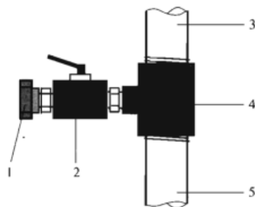
图 1 液阻和系统密闭性检测口示意
