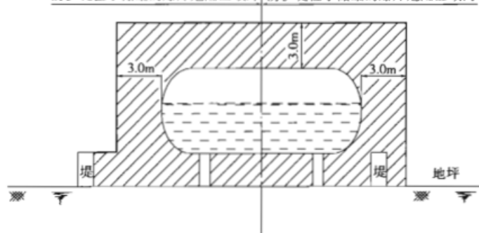
图 C.0.17-1 地上 LNG 储罐的爆炸危险区域划分
