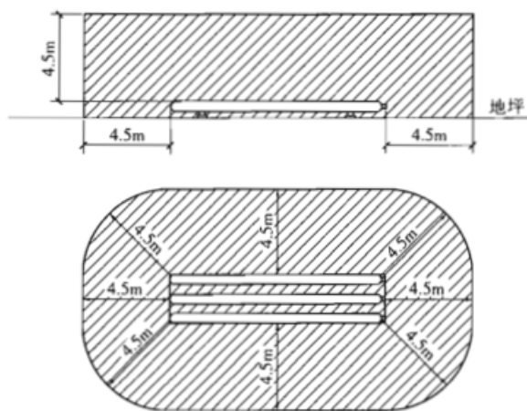
图 C. 0. 22 室外储氢容器的爆炸危险区域划分
