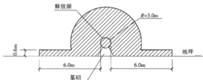
图 C.0.10 露天或棚内设置的 LPG 泵、压缩机、阀门、法兰或类似附件的爆炸危险区域划分
