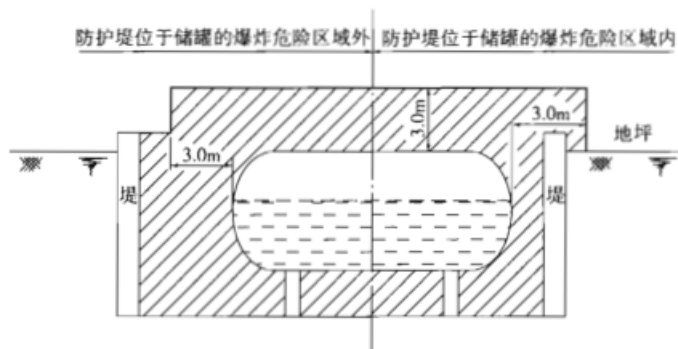
图 C.0.17-3 地下 LNG 储罐的爆炸危险区域划分
