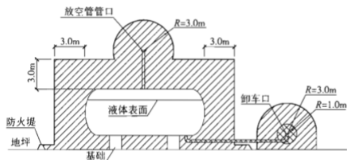
图 C.0.9 地上 LPG 储罐的爆炸危险区域划分
