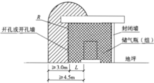
图 C.0.15 存放 CNG 储气瓶(组)房间的爆炸危险区域划分
