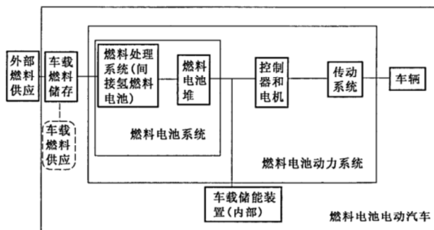
图 1 燃料电池电动汽车系统框图
