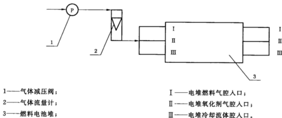
图3 气体气密性检查方法示意图
