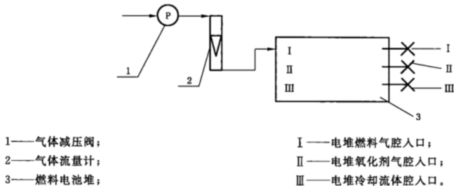
图 2 气体泄漏测试方法示意图
