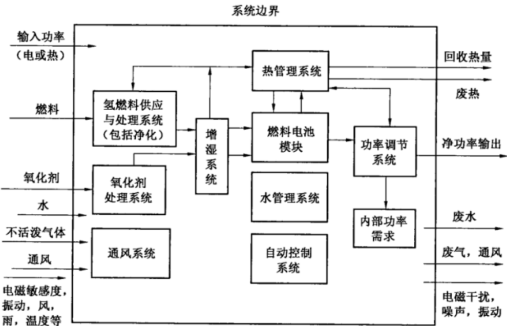
图1 发电系统的边界示意图
