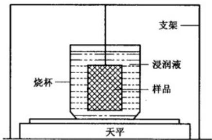
图 2 双极板密度测试装置示意图
